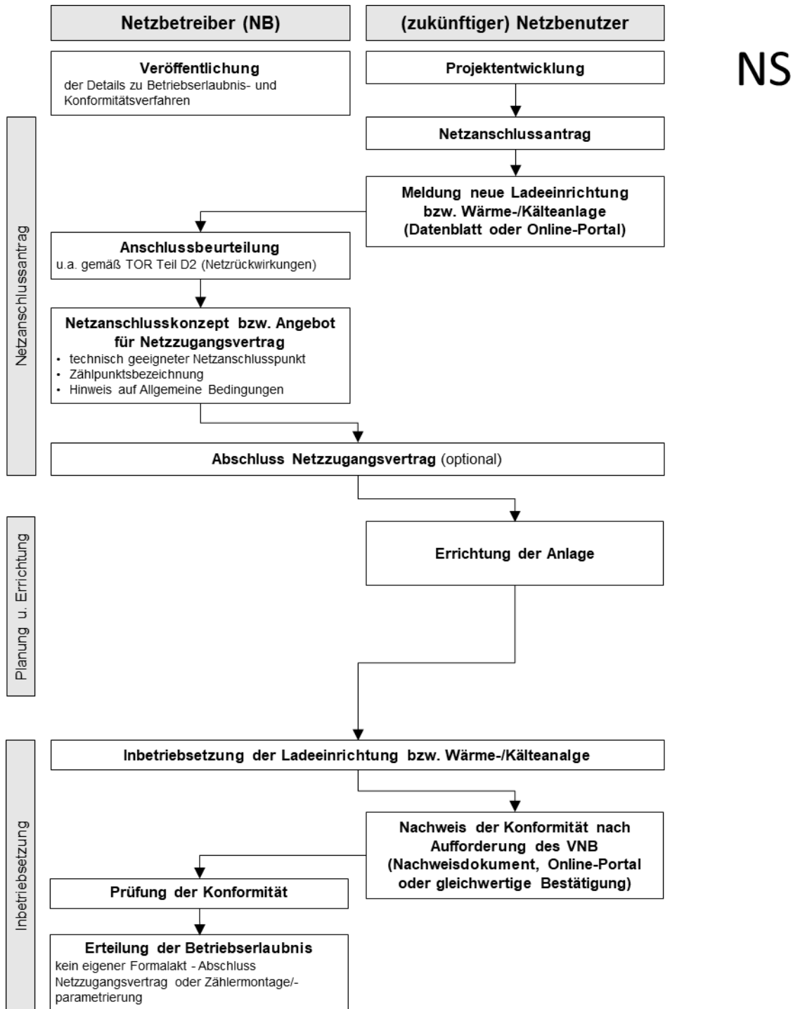
Abbildung 6: Ablauf des Betriebserlaubnisverfahrens für Ladeeinrichtungen und Wärme-/Kälteanlagen in der Niederspannung
