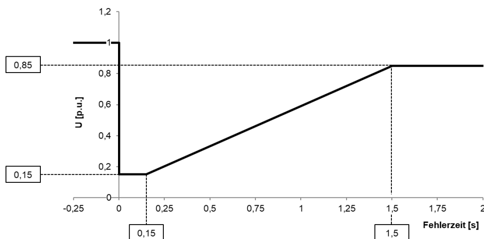
Abbildung 5: FRT-Profil mit Netzanschlusspunkt auf NS-Ebene
