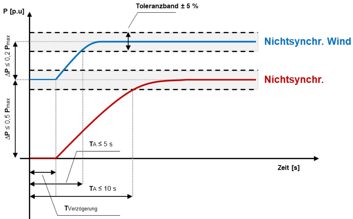
Abbildung 6: Beispiel für Anschlagzeiten nicht-synchroner Stromerzeugungsanlagen im LFSM-U Modus
