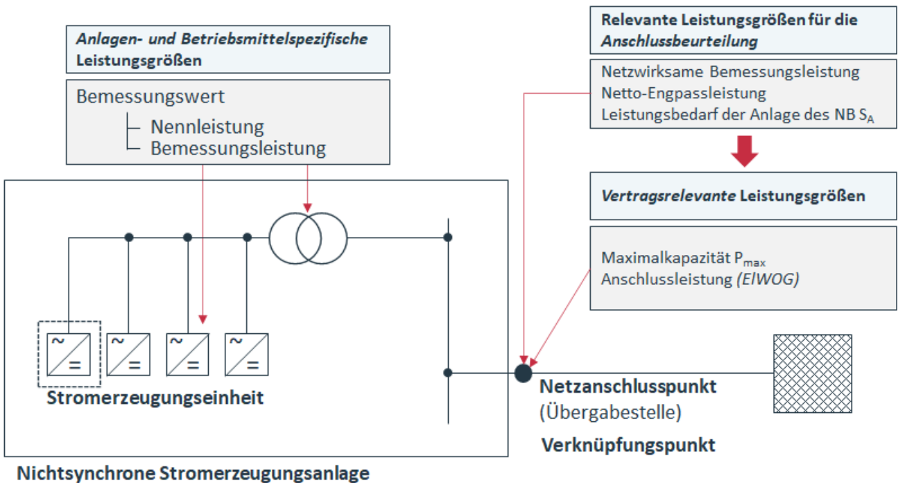
Abbildung 6: Schema Leistungsbegriffe nichtsynchrone Stromerzeugungsanlagen
