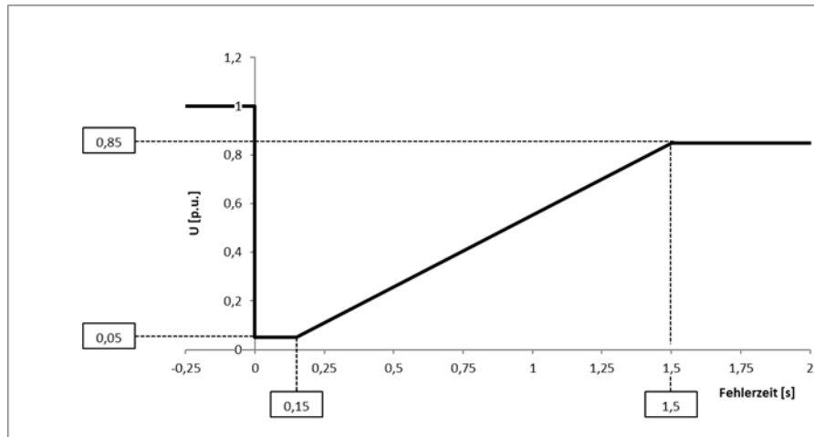
Abbildung 9: FRT-Profil nichtsynchrone Stromerzeugungsanlagen
