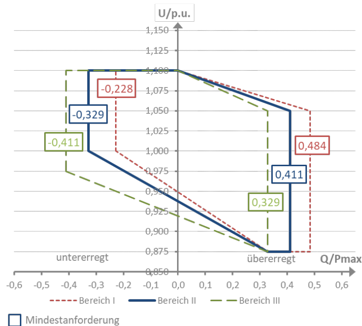
Abbildung 10: Blindleistungsbereiche synchroner und nichtsynchrone Stromezeugungsanlagen bei Maximalkapazität
