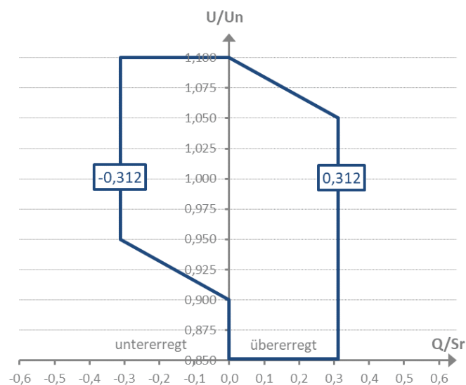
Abbildung 7: Blindleistungsbereich von Stromerzeugungsanlagen mit S_r \leq 3,68 kVA (ohne Umrichter 15 ) bei Nennscheinleistung
