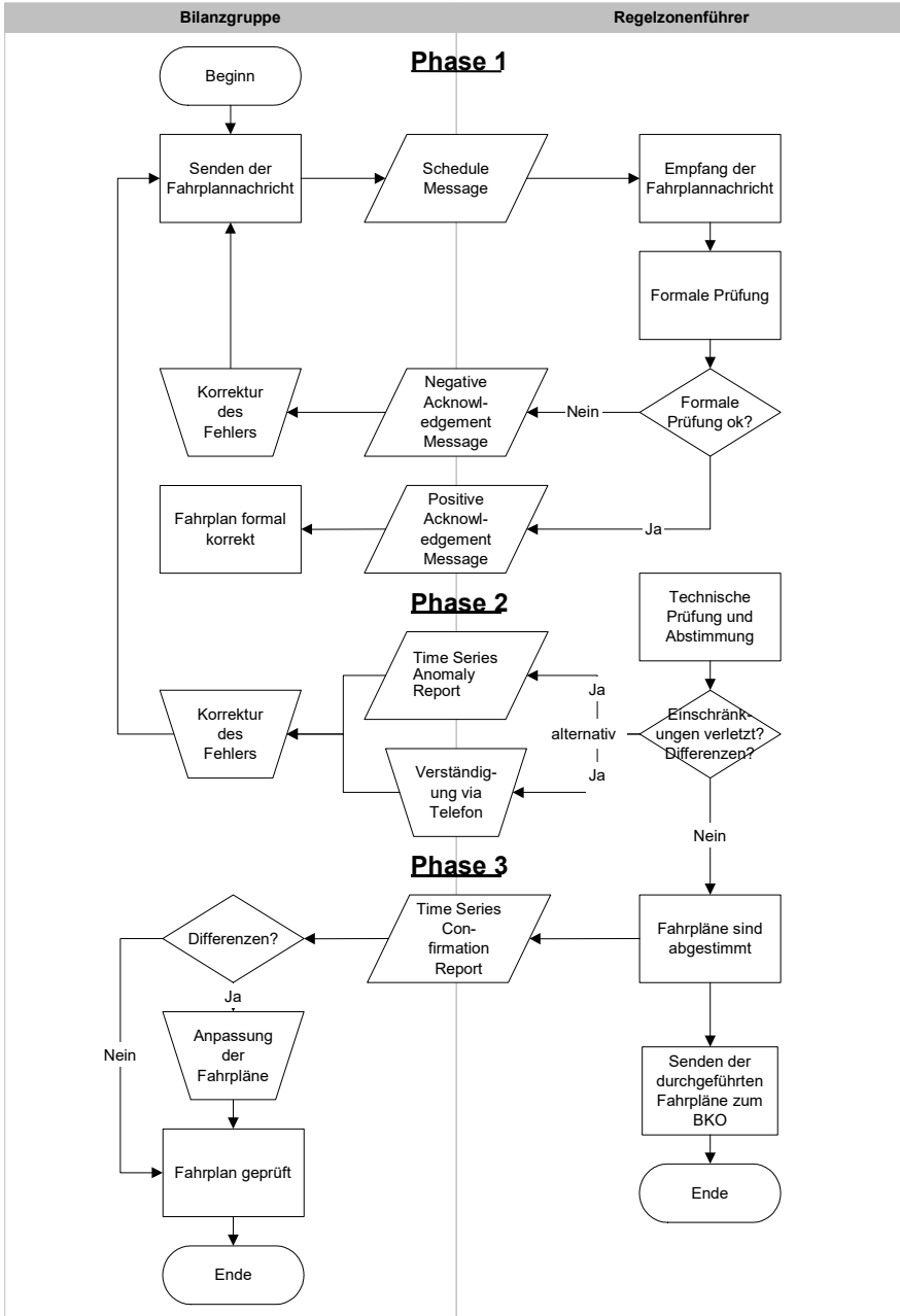
Abbildung 1: Meldung, Prüfung und Bestätigung externer Fahrpläne
