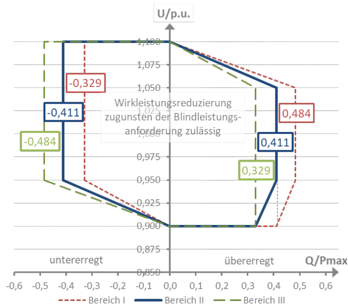
Abbildung 6: Blindleistungsbereiche synchroner und nichtsynchrone Stromezeugungsanlagen bei Maximalkapazität
