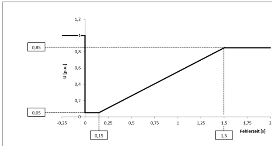
Abbildung 5: FRT-Profil nichtsynchrone Stromerzeugungsanlagen
