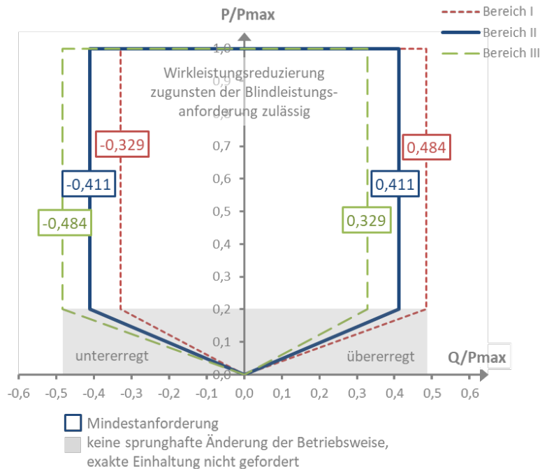
Abbildung 7: Blindleistungsbereiche synchroner und nichtsynchrone Stromezeugungsanlagen unterhalb der Maximalkapazität
