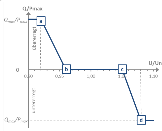
Abbildung 9: Blindleistungs-/Spannungskennlinie Q(U) im Niederspannungsnetz
