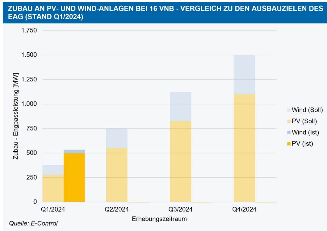
Abbildung 1: Entwicklung des Zubaus von Photovoltaik- und Windkraftanlagen ab 2024 bei 16 VNB im Vergleich zu den Ausbauzielen des EAG, Stand Q1 2024
