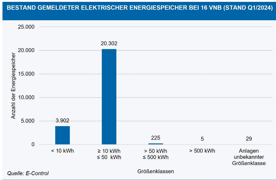
Abbildung 17: Bestand gemeldeter elektrischer Energiespeicher bei 16 VNB, Stand Q1 2024
