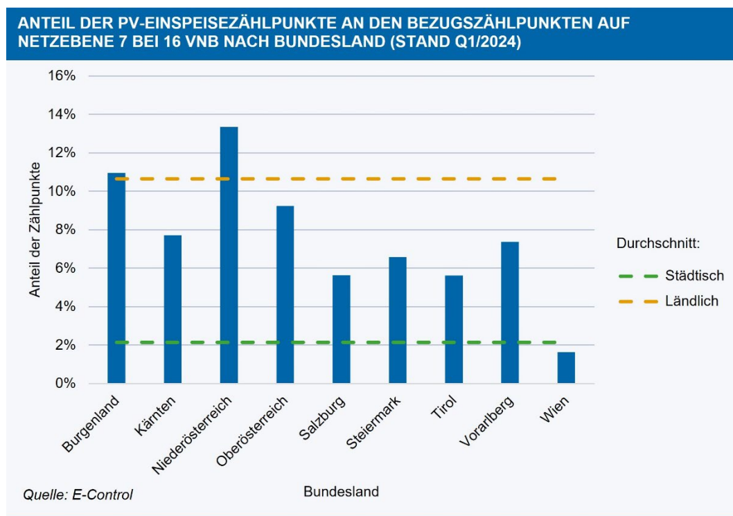
Abbildung 15: Anteil der Zählpunkte (Netzebene 7) für Photovoltaikanlagen an den Bezugszählpunkten bei 16 VNB in Q1 2024
