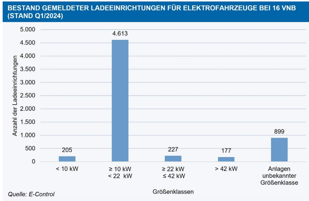
Abbildung 18: Bestand gemeldeter Ladeeinrichtungen für Elektrofahrzeuge bei 16 VNB, Stand Q1 2024
