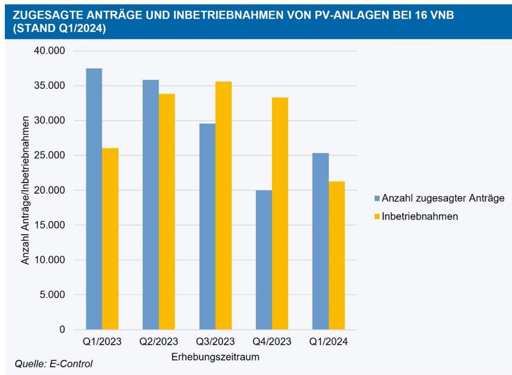
Abbildung 7: Zugesagte Anträge und neue Inbetriebnahmen von Photovoltaikanlagen bei 16 VNB ab 2023, Stand Q1 2024
