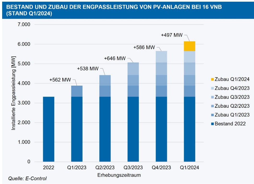
Abbildung 2: Entwicklung des Bestands und des Zubaus von Photovoltaik ab 2022 bei 16 VNB, Stand Q1 2024
